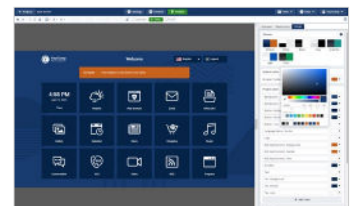
Fig. 3: Customizable templates
