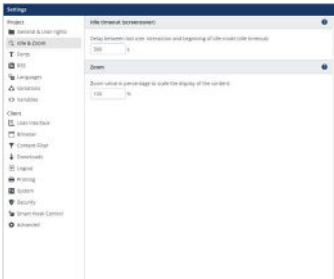
Fig. 3: Screensaver options
